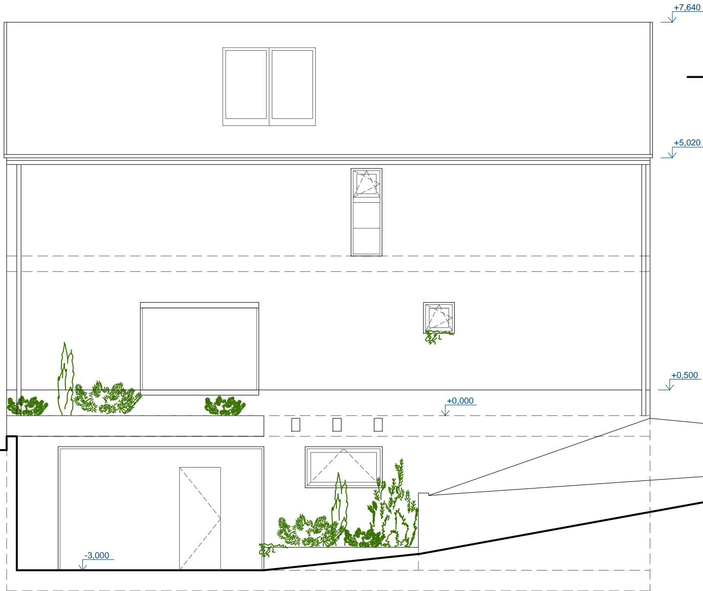
ZÁPADNÍ POHLED
